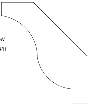
CW527W 1 9/32"W x 2"H
